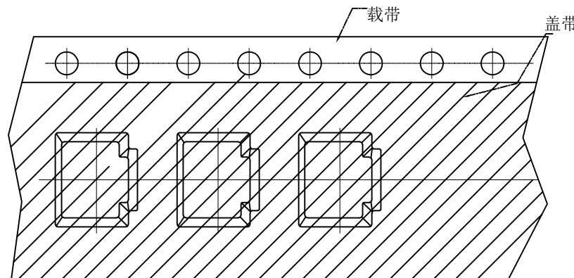
包装图
