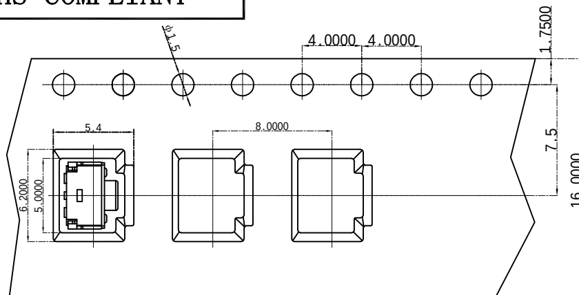
载带尺寸图
