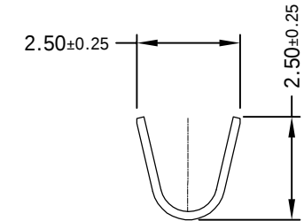
SEC: A-A
